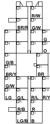
X-17 中部线束 (M) - 前门线束右 (DR2)
