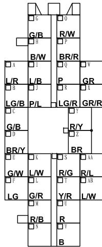
X-16 中部线束 (M) - 前门线束左 (DR1)
